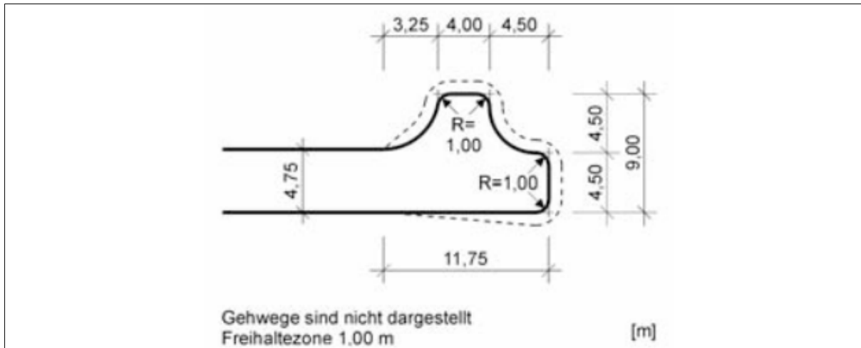
Abbildung 1: Auszug RAS 06 FGSV Verlag; Flächenbedarf für einen Wendehammer für Pkw
