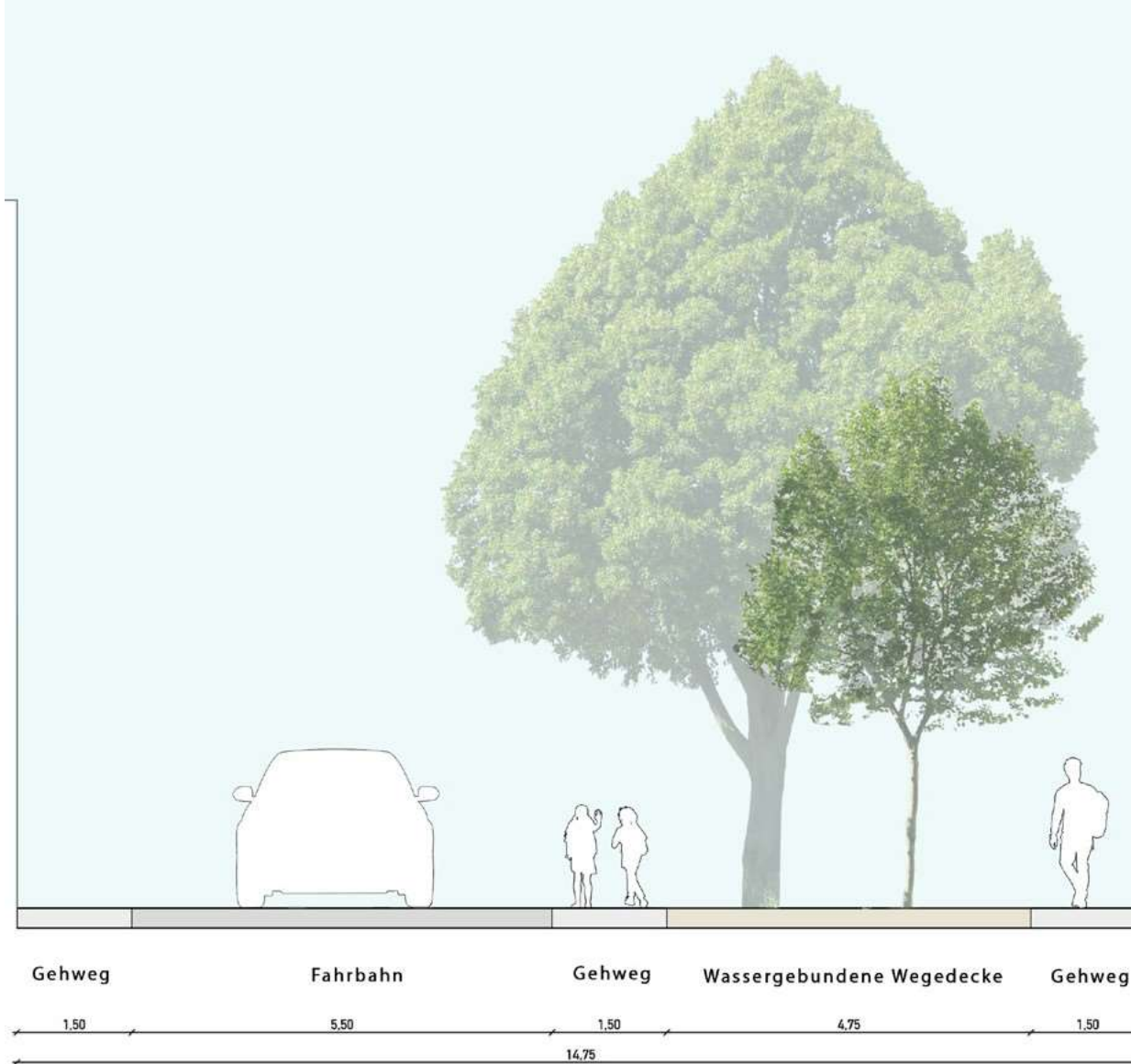
Abbildung 56: Straßenquerschnitt Goebenstraße.
