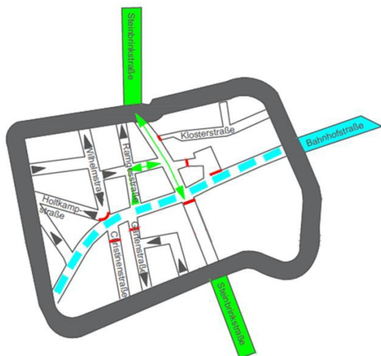
Abb.7: Verkehrsbeziehung nach Umsetzung der Maßnahmen
