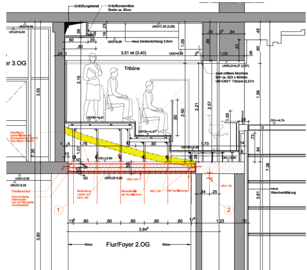
Schnitt A-A Tribüne
