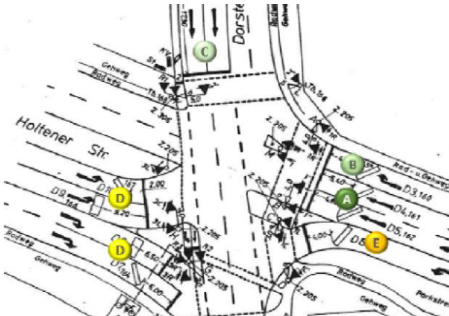
Abbildung 1: Knotenpunkt Dorstener Straße / Teutoburger Straße: Verkehrsqualitäten der einzelnen Fahrbeziehungen im Bestand nach HBS 2001 (A = Sehr gut - F = ungenügend)
