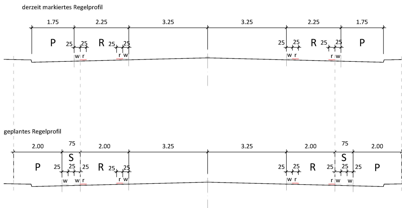
Abbildung 1: Derzeitiges und geplantes Regelprofil
