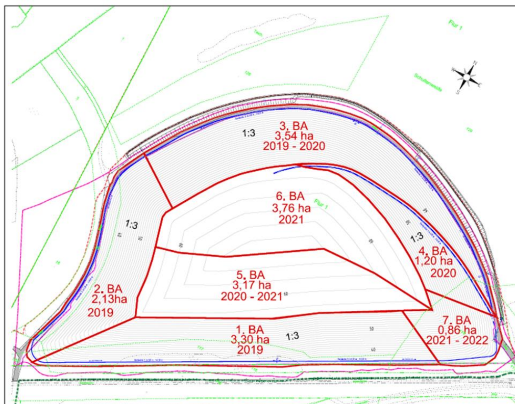
Abb. 2: Lageplan Bauphasen/ Bauzeitenplan, M. 1:2.000
