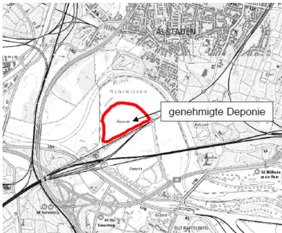
Abb. 1: Übersichtslageplan der Deponie Kolkerhofweg in Mülheim an der Ruhr
