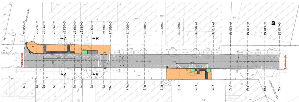
Abbildung 1: Lageplan der Straßenbauplanung mit Darstellung der Haltestellenbereiche (WBO GmbH)
