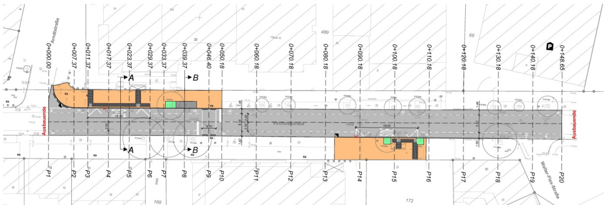
Abbildung 1: Lageplan der Straßenbauplanung mit Darstellung der Haltestellenbereiche (WBO GmbH)
