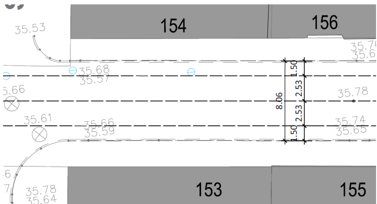
44 45 Abbildung 1: Beidseitig Schutzstreifen
