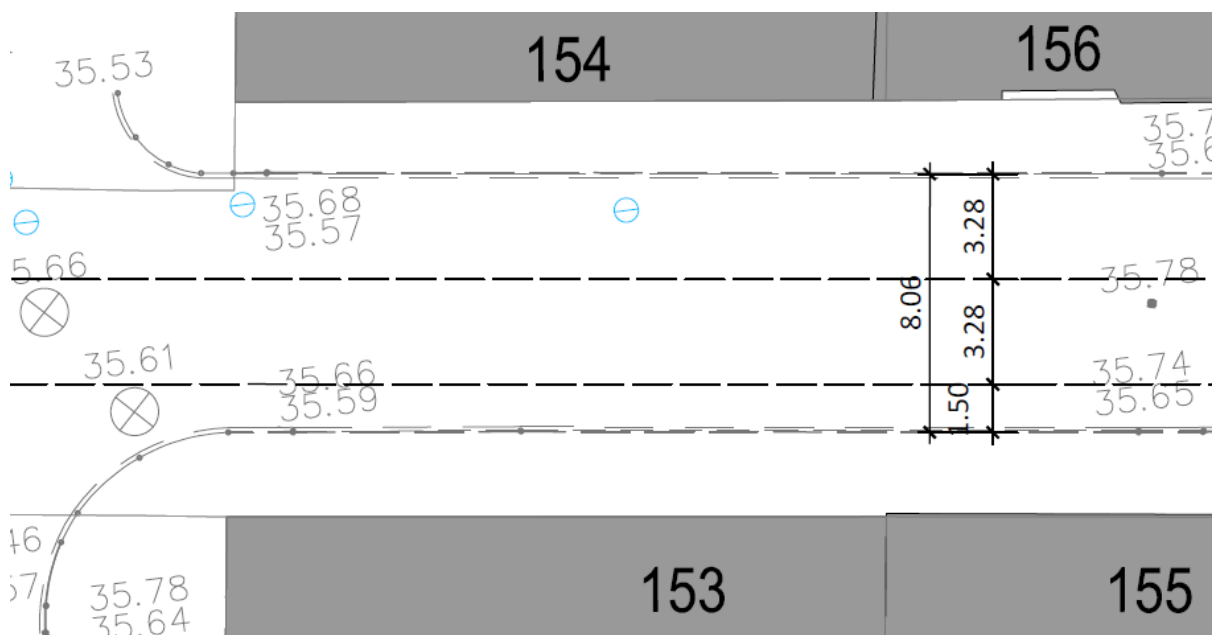
54 55 Abbildung 2: Einseitiger Schutzstreifen
