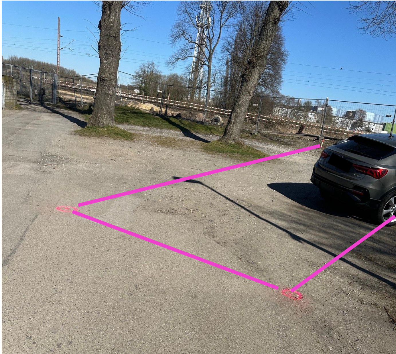
Markierung der Startgrube
