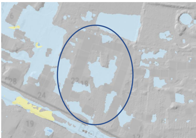
Abbildung 8: Starkregengefahrenkarte NRW
