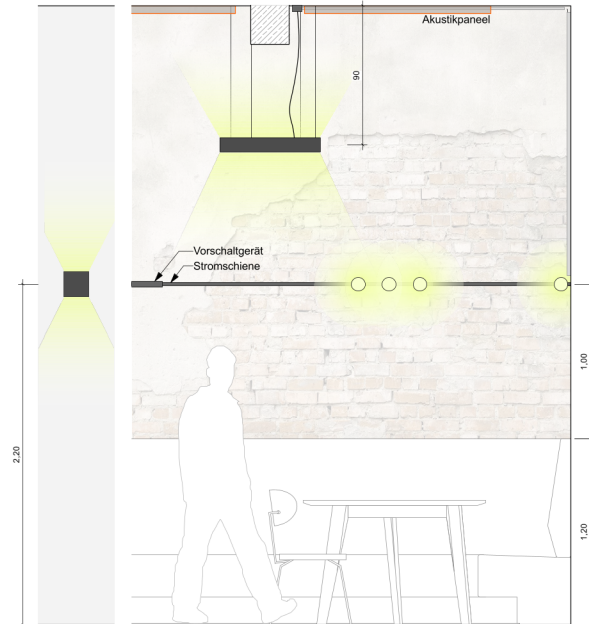
Schemadetail Beleuchtung Gastraum | 1:20
