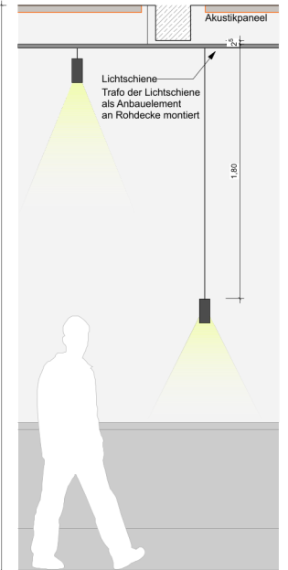
Schemadetail Beleuchtung Theke | 1:20
