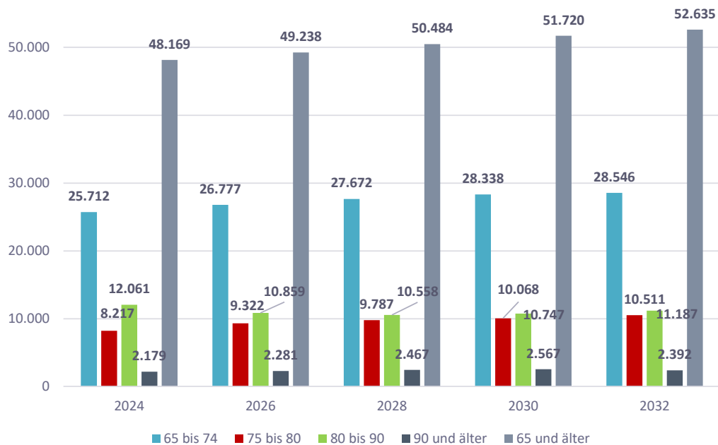
ALTERSGRUPPEN PROGNOSE
