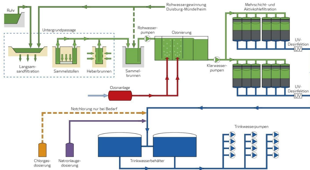
Abbildung 10: Verfahrensfließbild Wasserwerk Mülheim-Styrum/Ost
