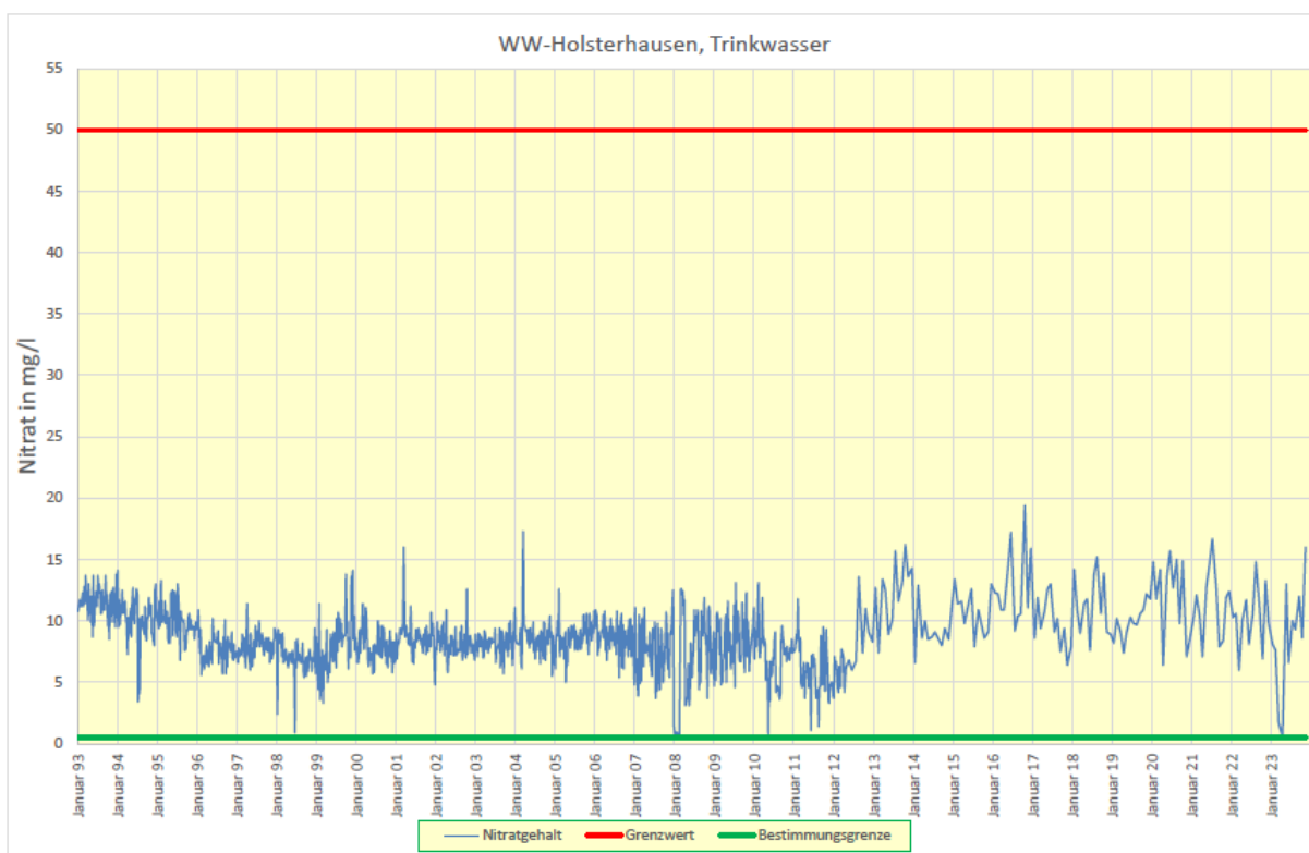
Abbildung 19: Nitratkonzentration im Trinkwasser des Wasserwerks Holsterhausen
