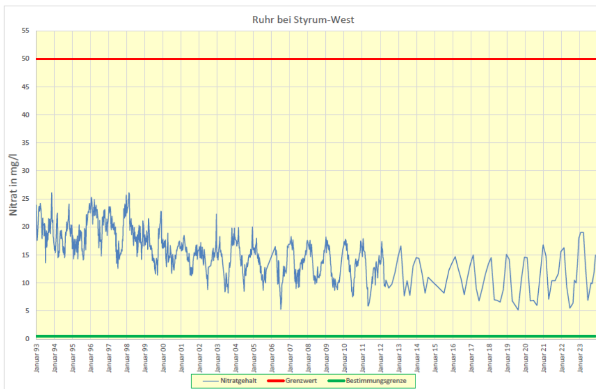
Abbildung 14: Nitratkonzentration in der Ruhr bei Mülheim Styrum West
