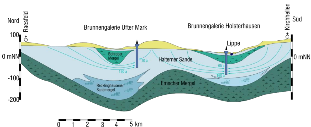
Abbildung 9: Schematisches geologisches N-S-Profil durch das Wassergewinnungsgebiet
