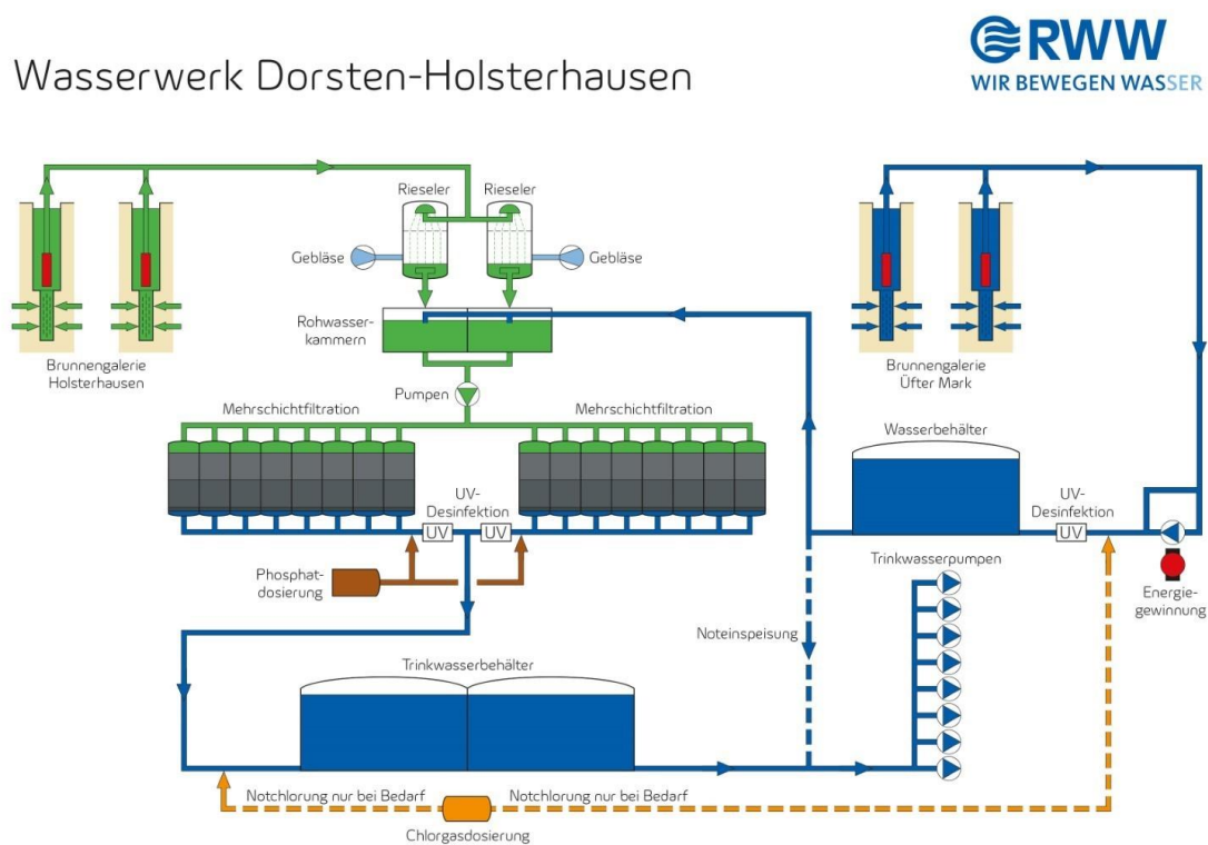
Abbildung 7: Verfahrensfließbild Wasserwerk Dorsten-Holsterhausen
