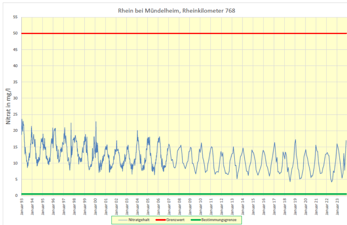
Abbildung 16: Nitratkonzentration im Rhein bei Duisburg-Mündelheim
