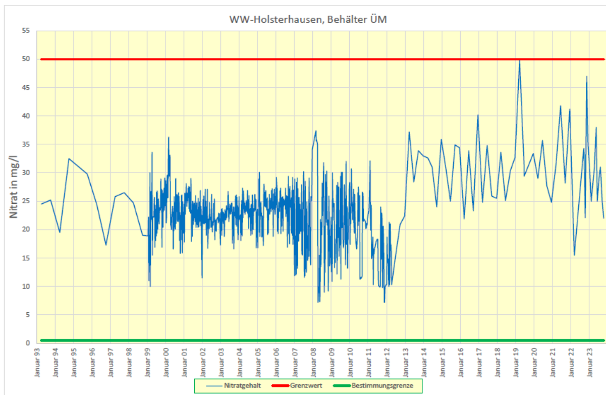
Abbildung 18: Nitratkonzentration im Rohwasser der Brunnengalerie Üfter Mark
