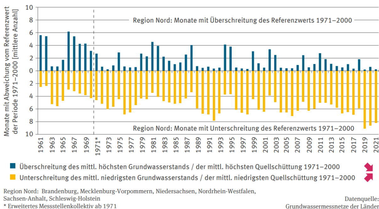
Abbildung 20: Grundwasserstand und Quellschüttung in der Region Nord
