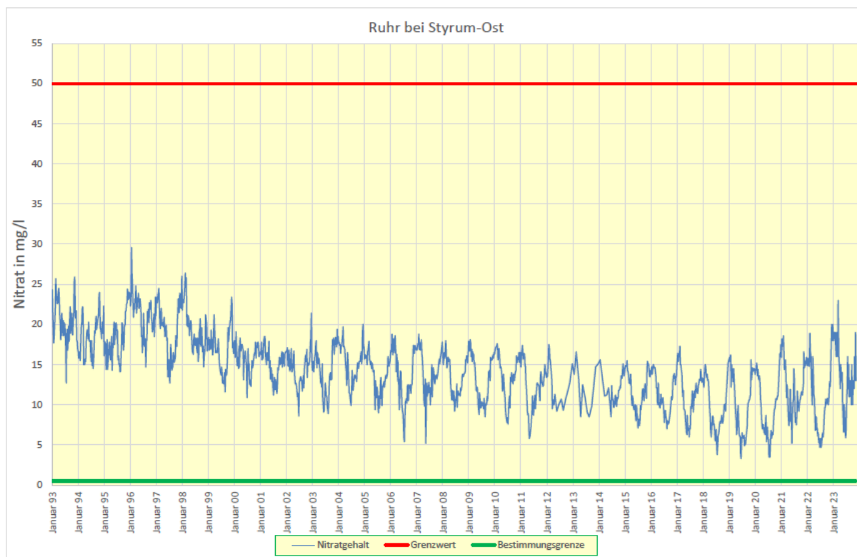
Abbildung 15: Nitratkonzentration in der Ruhr bei Mülheim Styrum Ost
