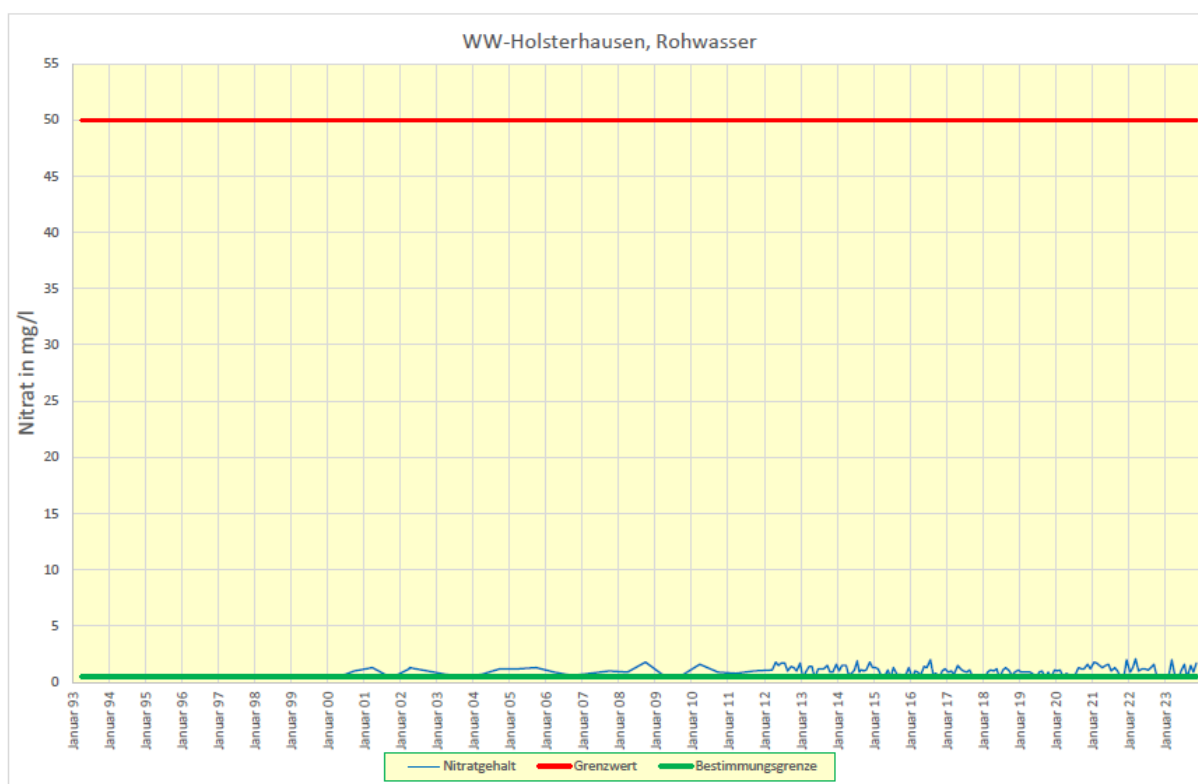
Abbildung 17: Nitratkonzentration im Rohwasser der Brunnengalerie Holsterhausen
