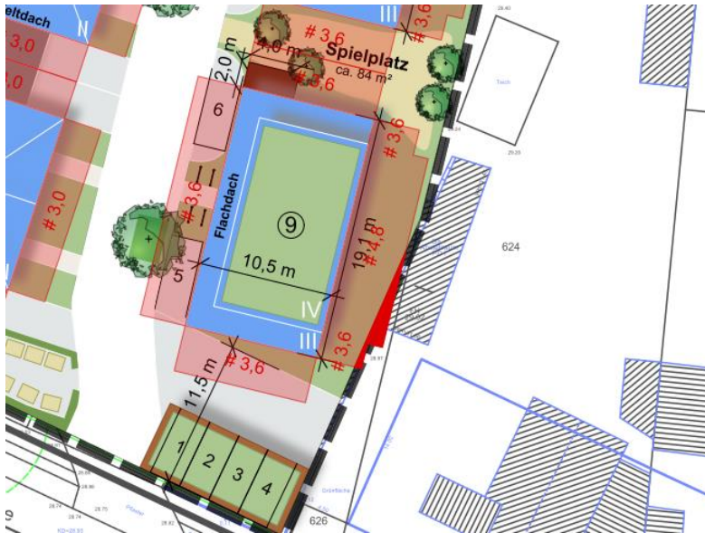
Abbildung 7: Überschreitung der Abstandsflächen gem. § 6 Abs. 5 BauO NRW
